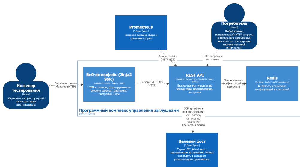
Рисунок 2 – Контейнерная диаграмма системы (C4 Level 2)
